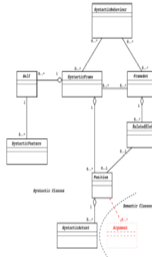
FIG. 5 – Extension syntaxique de LMF
