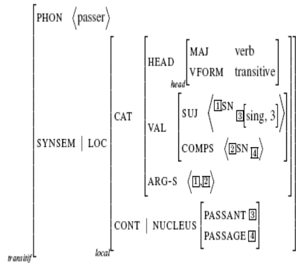
FIG. 1 – Entrée lexicale du verbe passer
